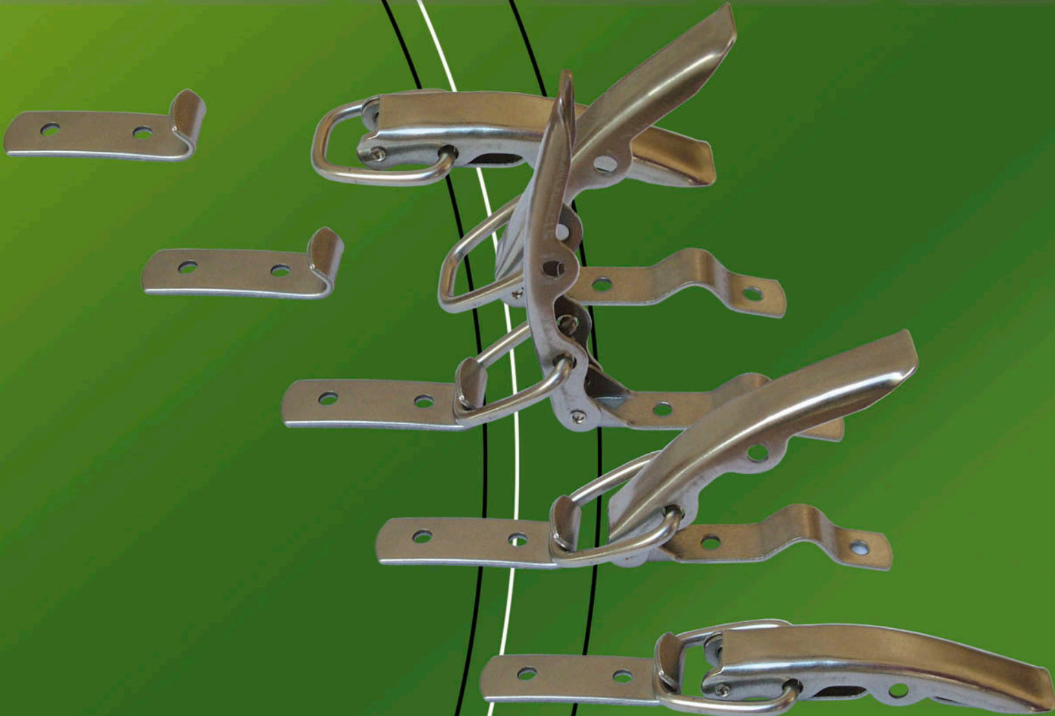
Art. nr. C 15-20 BLSH=15/50/2,0/12 A2 Catch plate Békázár ellendarab
